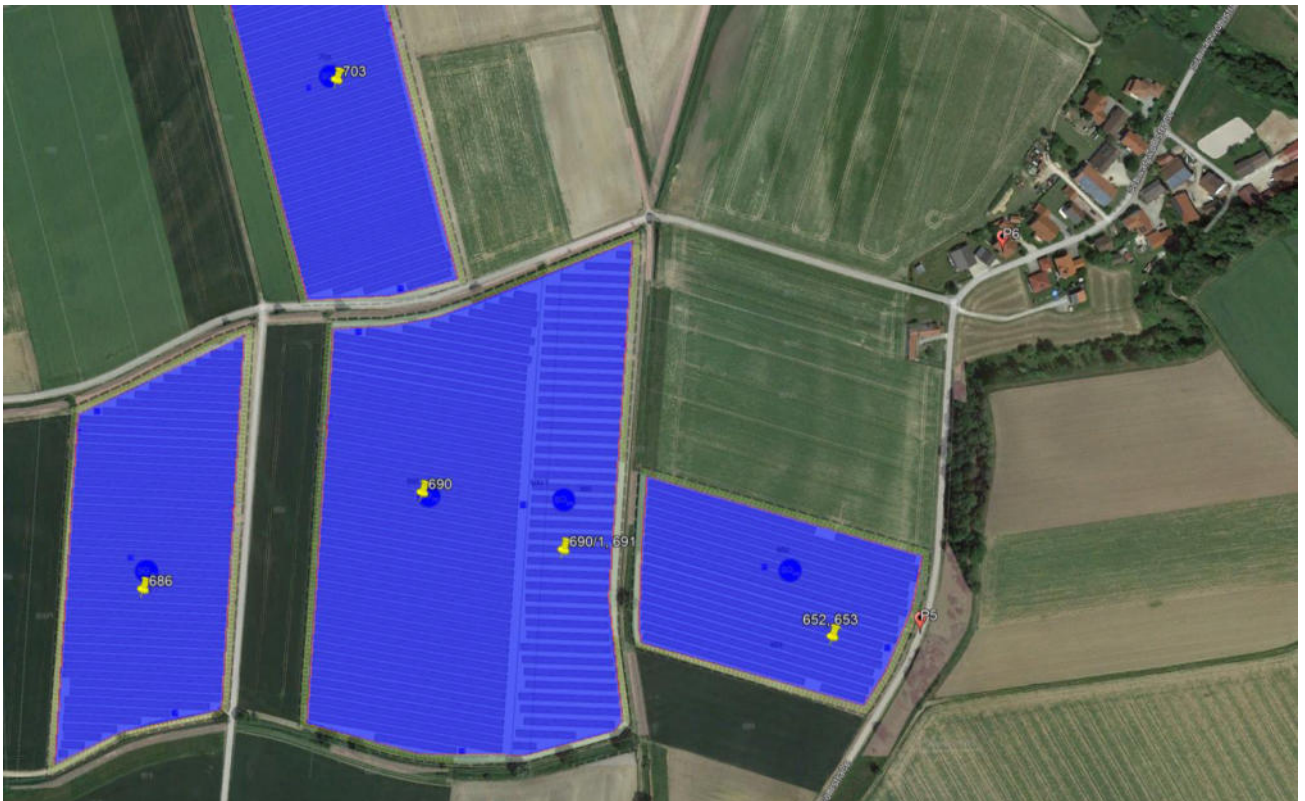
Bild 3.5.3: Übersicht über die PV-Anlage Ost und die Messpunkte (Quelle: Google Earth/SolPEG)
