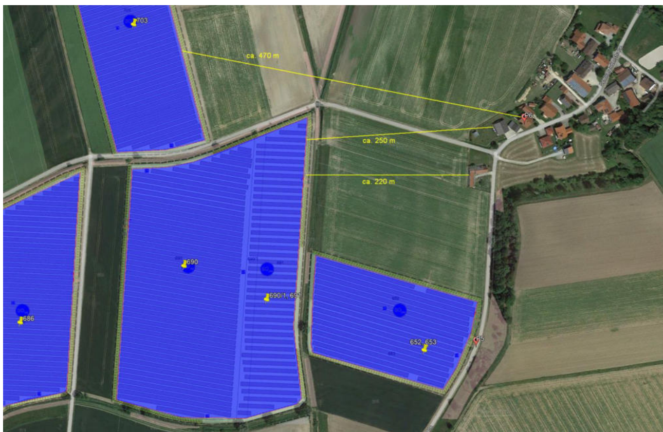
Bild 4.6.1: Entfernungen zu den PV-Flächen (Quelle: Google Earth/SolPEG)
