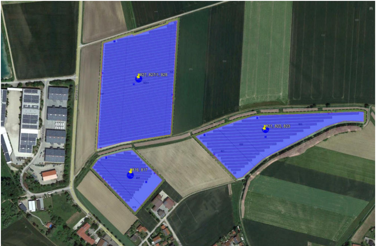
Bild 2.1.4. Detailansicht der PV-Fläche Teil Nord (Quelle: Google Earth/SolPEG)
