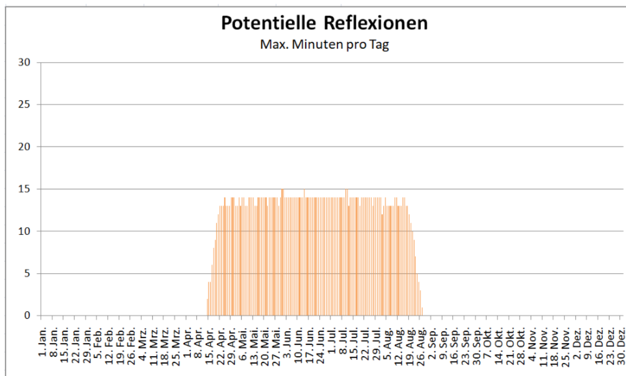
Bild 4.4.1: Reflexionen pro Tag im Jahresverlauf am Messpunkt P1 (Quelle: Simulationsergebnisse, aufbereitet)
