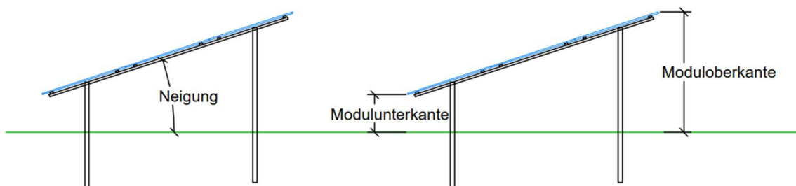
Abbildung 3.3: Skizze Modultisch
